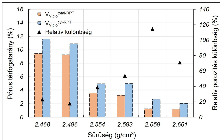
14. ábra: A mért porozitás ( V_v ) és a relatív porozitás különbségek ( \Delta_{rel} V_v ): a vizsgált térfogat változásának hatása ( ^{vol-eff, RPT} ) ([8] nyomán).
