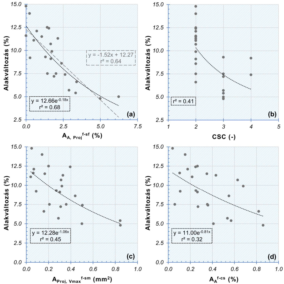
26. ábra: A regressziós modellezéssel meghatározott, az alakváltozást ( \varepsilon (%)) leginkább befolyásoló pórusjellemzők diagramjai: (a) A_{A, Proj}^{f-sf} (0–6,23% között), (b) CSC, (c) A_{Proj, Vmax}^{f-sm} (0,04–0,85 mm 2 között) és (d) A_A^{f-cs} (0,04–0,86% között) [12].
