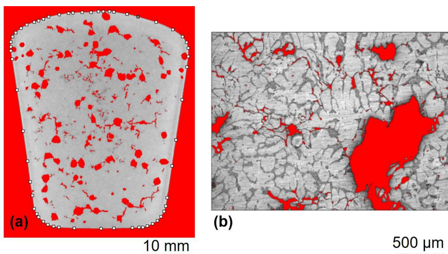
9. ábra: Az ImageJ képelemzővel történt 2D-s elemzések: (a) a teljes próbatest hosszirányú sorozatmetszeteinek ( A_{A, CT}^{\text{total-RPT}} ) és (b) a teljes próbatest közép-hosszsmetszetéről készült mikroszkópos felvételeinek ( A_{A, OM}^{\text{total-RPT}} ) elemzése ([8] nyomán).
