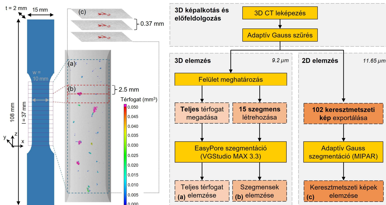
17. ábra: A szakító próbatetek méretei és a CT-felvételek elemzett régiói (az ábra bal oldalán), valamint a 3D-s és 2D-s képelemzési eljárások (az ábra jobb oldalán): (a) a teljes térfogat, b) a 15 szegmens, és c) a keresztmetszeti képek [12].
