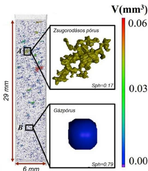
1. ábra: Szakító próbatestben méret (térfogat) és morfológia (gömböszerűség) alapján megkülönböztetett pórus [9].
