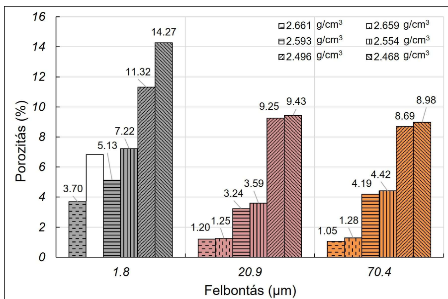
11. ábra: A különböző sűrűségű próbatestekben mért porozitás a vizsgálati módszerek felbontásának függvényében (az OM módszerrel mért 2,659 \text{ g/cm}^3 sűrűségű test porozitás értéke kiugró adat, ezért azt külön ábrázoltam) [8].
