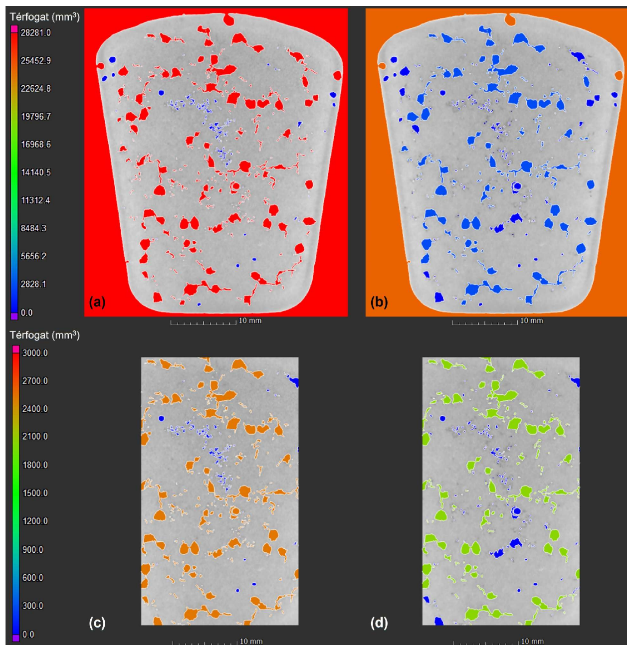
8. ábra: A vizsgált testek 3D-s elemzésének eredményei hosszsz metszeti ábrákon bemutatva: (a) morfológiai transzformáció (zárás) nélkül, felületre kifutó nyitott pórusokkal; (b) morfológiai transzformáció után zártak a pórusok; (c) a henger térfogat zárás nélkül; (d) a henger térfogat zárás után [8].
