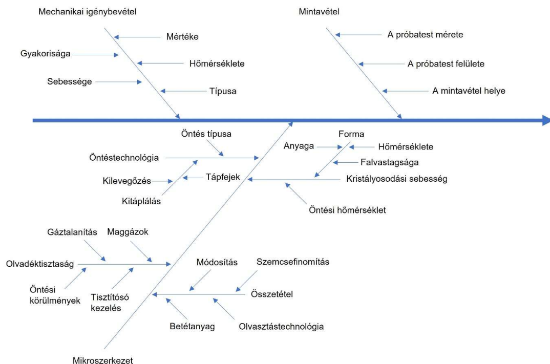
4. ábra: Az öntvények mechanikai jellemzőit befolyásoló tényezők [95].
