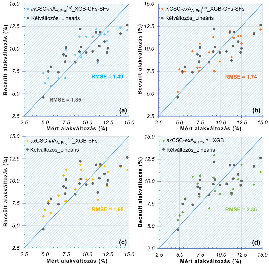
24. ábra: Az alakváltozás ( \epsilon (%)) mért és becsült értékeinek összehasonlítása a kiemelt jellemzők (CSC és A_{A, Proj}^{f-sf} ) egyes kombinációival felépített modellek esetén: (a) inCSC-inA_{A, Proj}^{f-sf} , (b) inCSC-exA_{A, Proj}^{f-sf} , (c) exCSC-inA_{A, Proj}^{f-sf} és (d) exCSC-exA_{A, Proj}^{f-sf} . Az ábrarészek tartalmazzák a lineáris kétváltozós (Kétváltozós_Lineáris) modellel becsült értékeket is [12].
