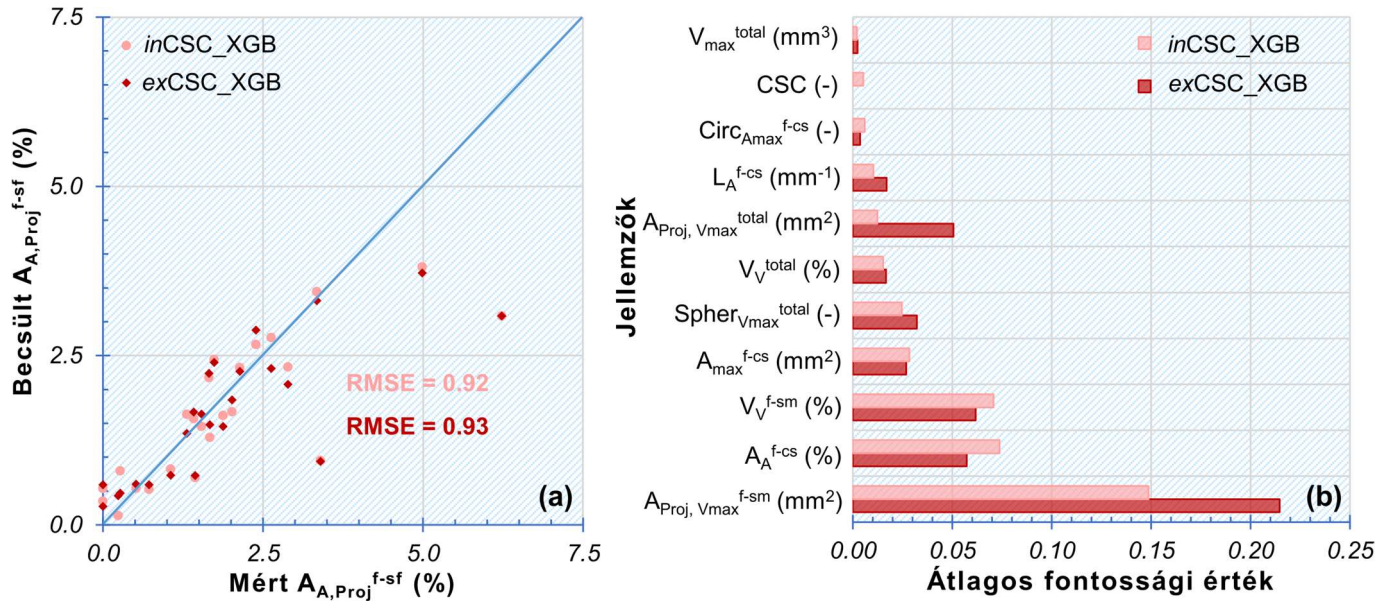
27. ábra: A töretfelületi porozitás ( A_{A, Proj}^{f-sf} (%) ) becslése a kiemelt CSC független változóval ( inCSC ), illetve nélkül ( exCSC ): (a) a mért és becslült értékek összehasonlítása, illetve (b) az egyes független változók fontossága a modellekben [12].
